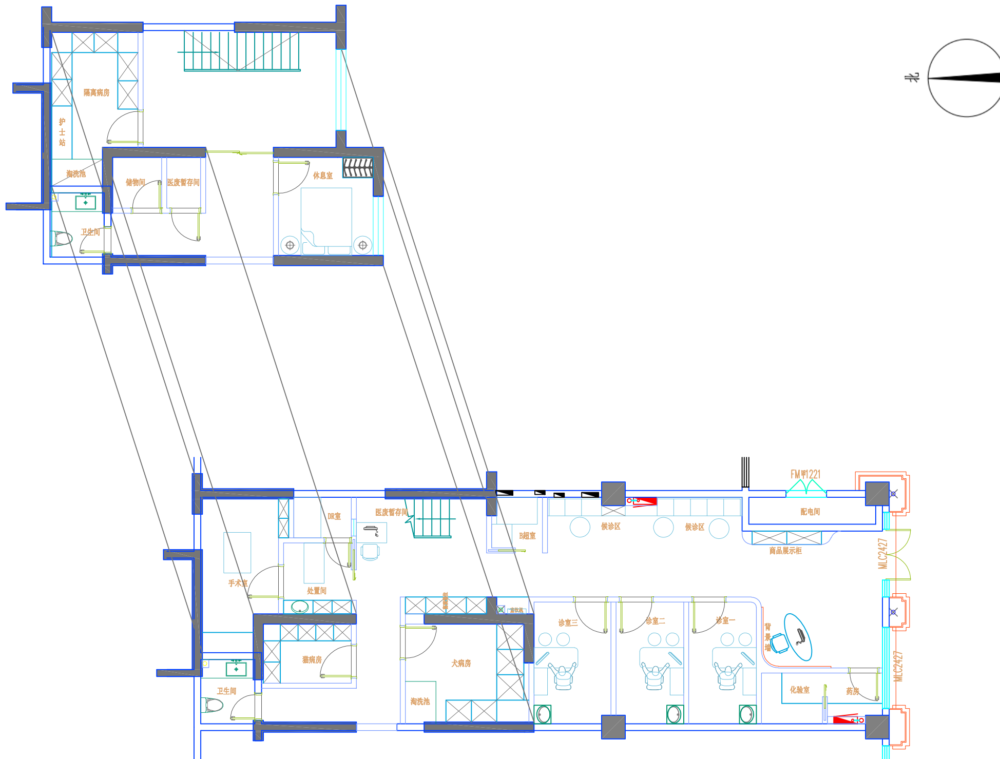
附图4 平面布置图
