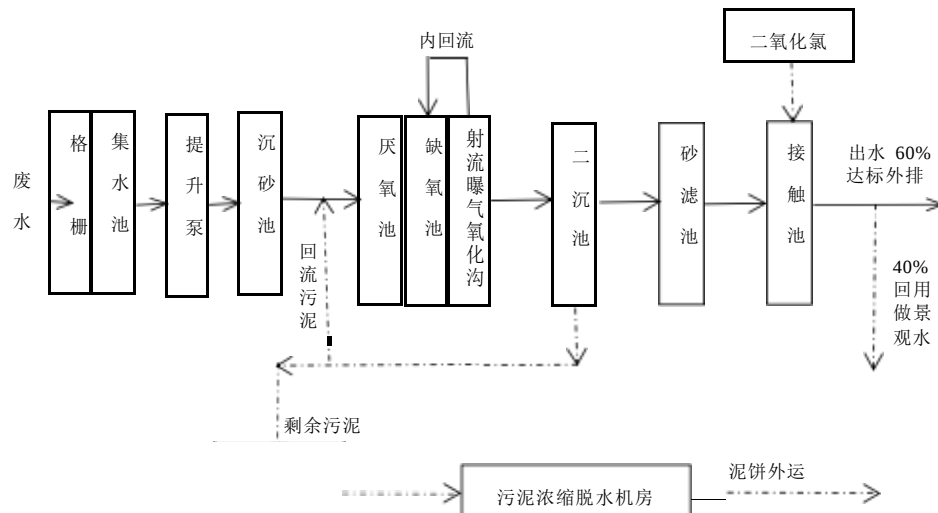
图 5 本项目校区污水处理站工艺流程
